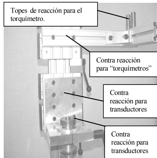
Figura 6. Sistema de contra reacción.
