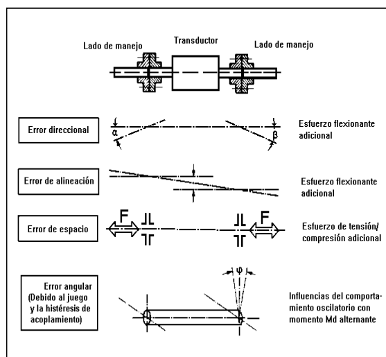
Figura 3. Errores en la instalación de instrumentos de medición de par torsional.
