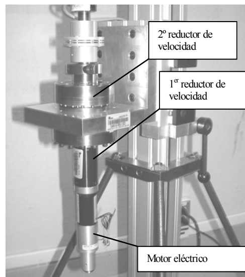
Figura 3. Subsistema para generación del par torsional.
